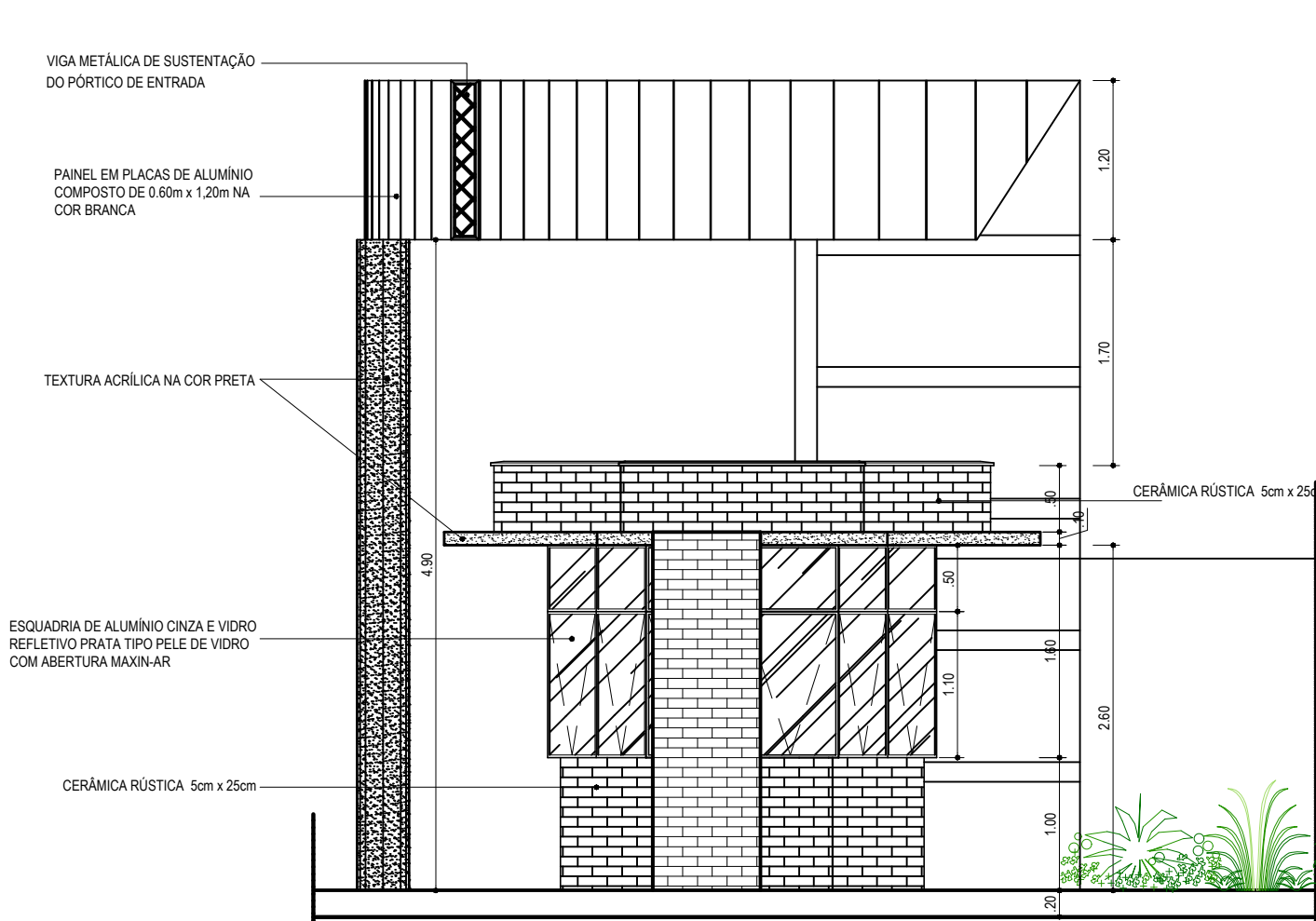
VISTA - 02 ESCALA.....1/50
