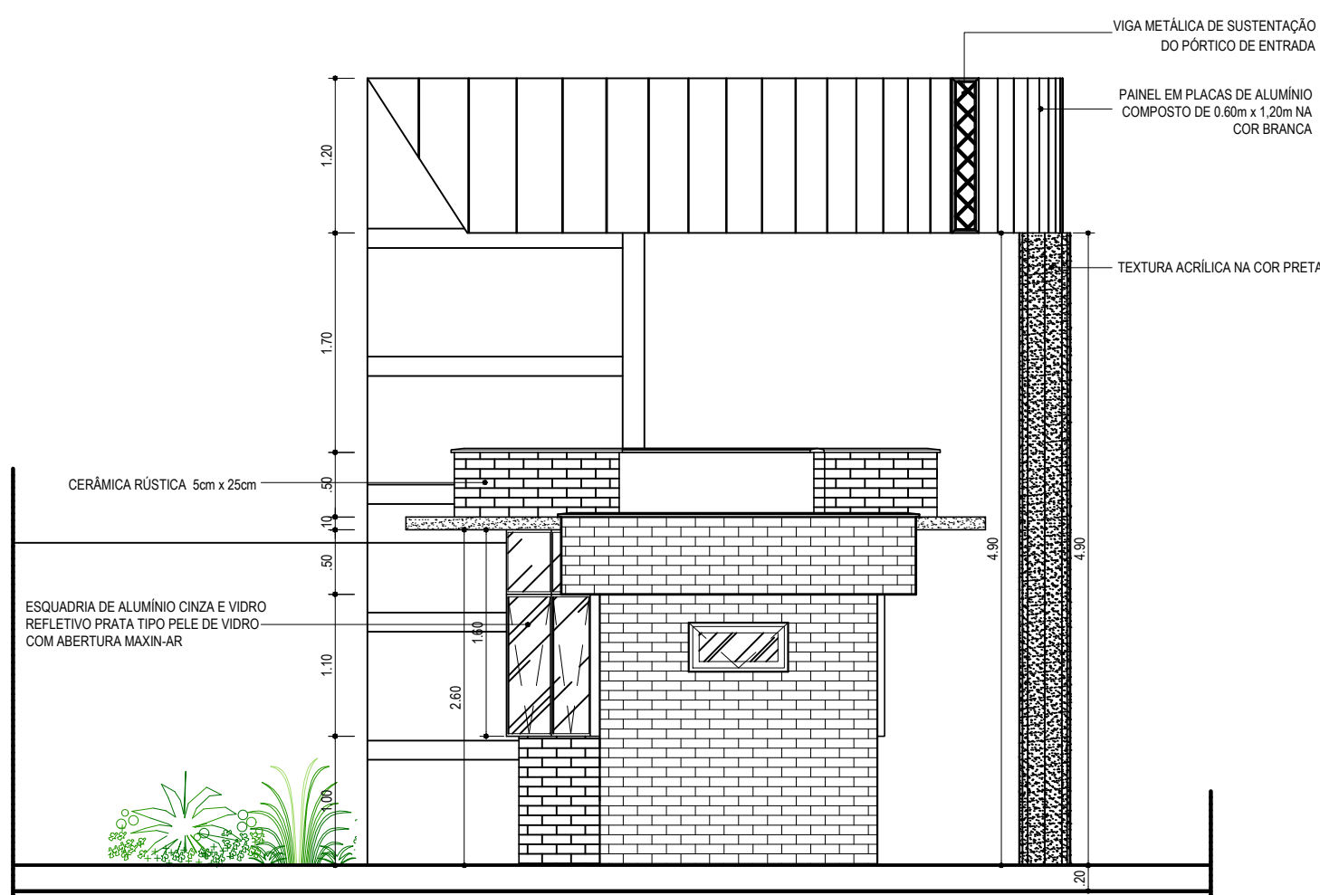
VISTA - 03 ESCALA.....1/50
