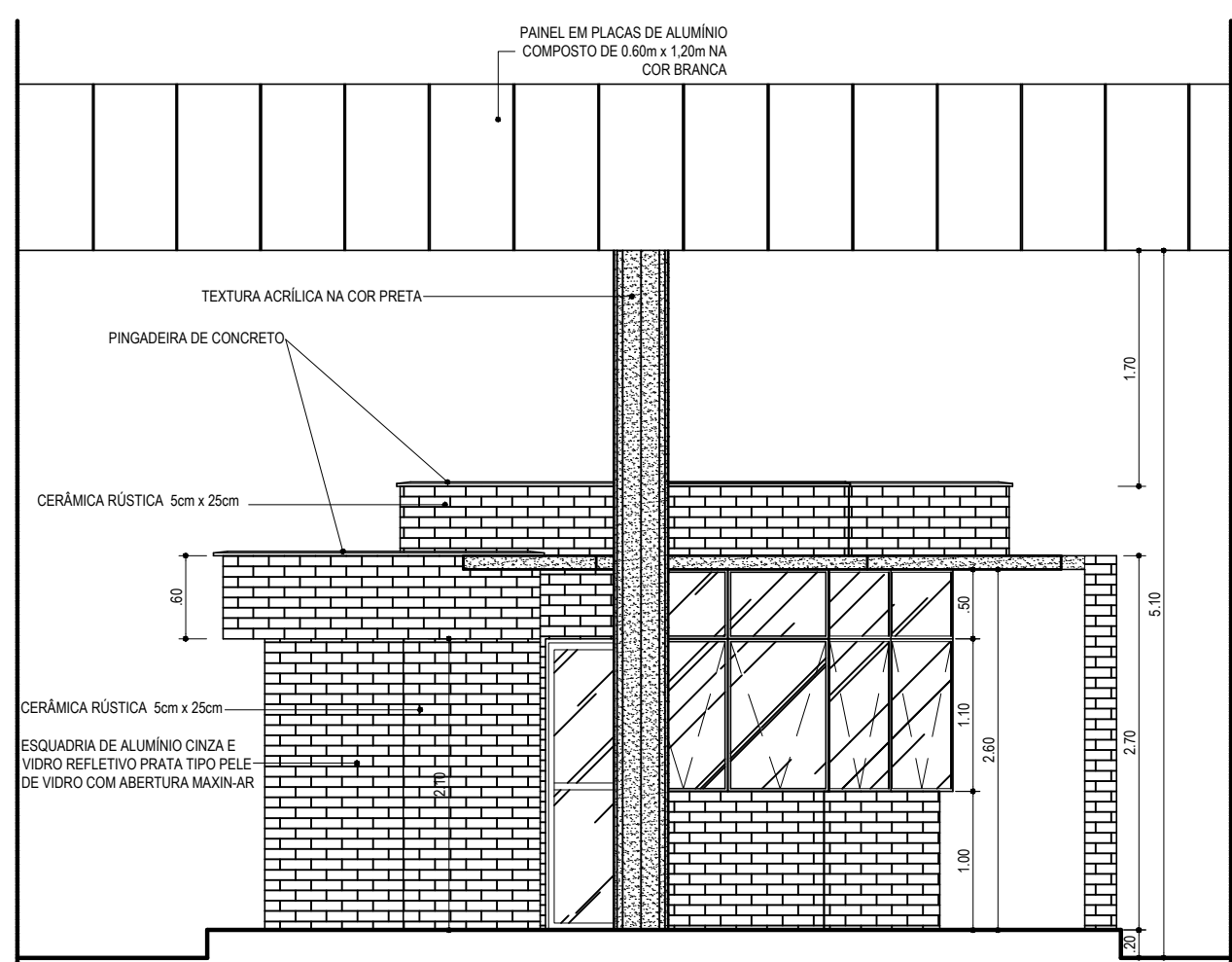
VISTA - 04 ESCALA.....1/50
