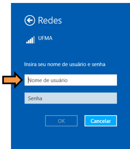
Figura 4 - Autenticação
