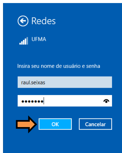
Figura 5 – Login
